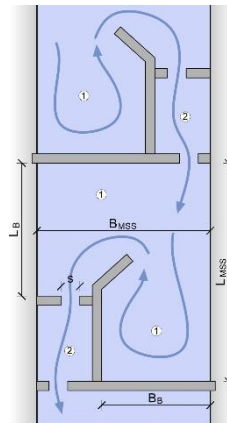
Systemskizze nach www.maba-fischpass.com (mod.) und A. Peter, aus BAFU (2022)
