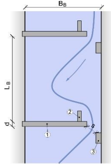
Systemskizze nach DWA 2014 (mod.) und M. Mende, aus BAFU (2022)
