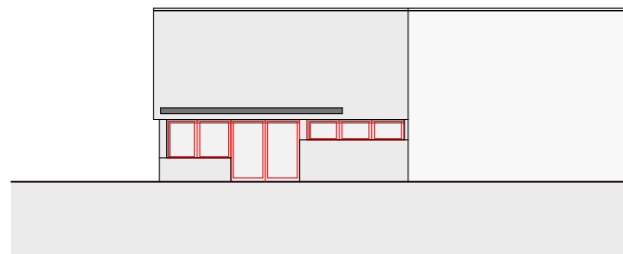
Ostfasade
