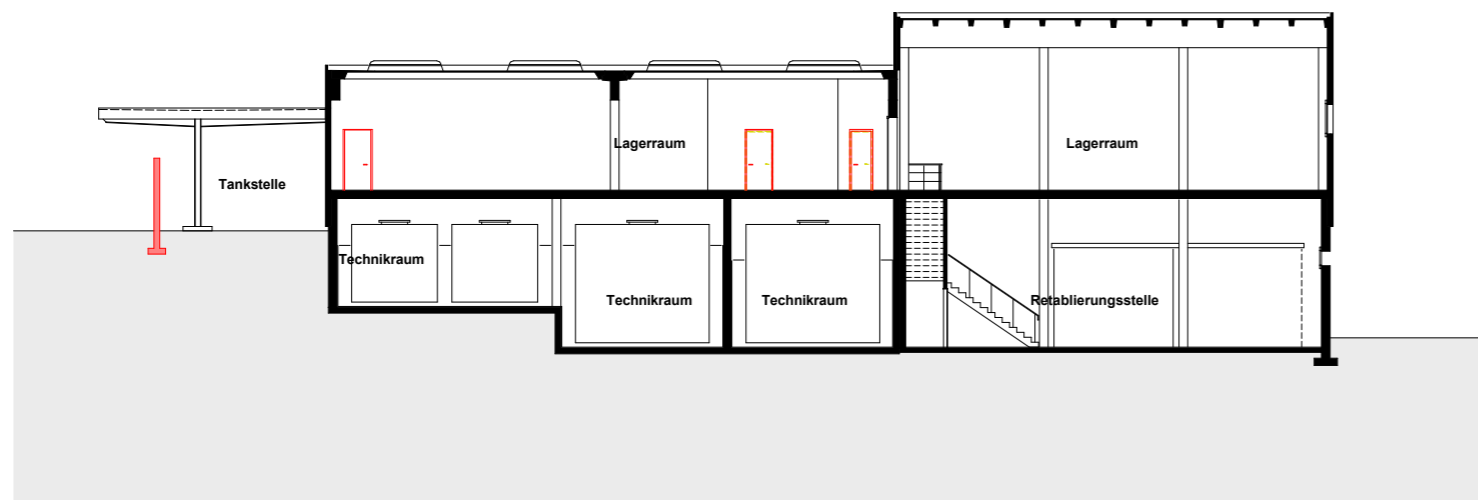
Querschnitt A-A
