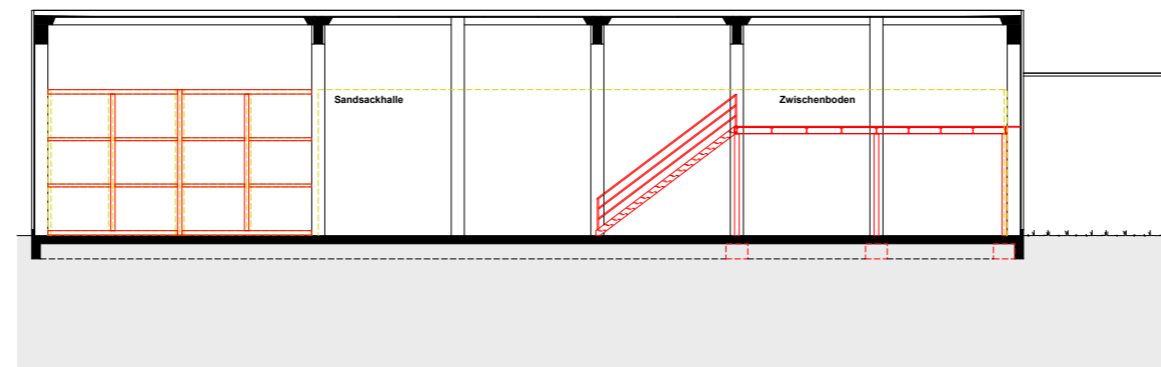
Querschnitt A-A
