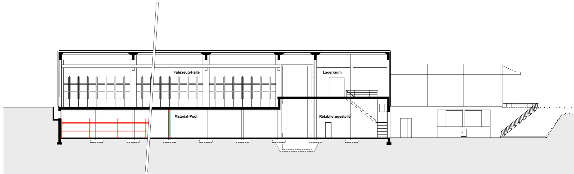
Längsschnitt B-B
