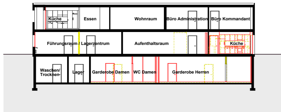
Querschnitt A-A
